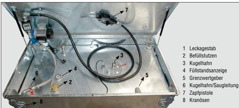
Typ MT 1000 mit Elektropumpe (Zubehör)
