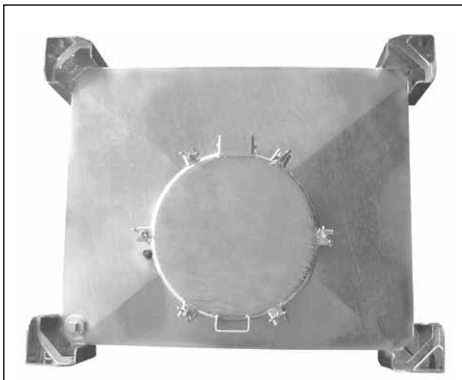
versetzter Domdeckel
