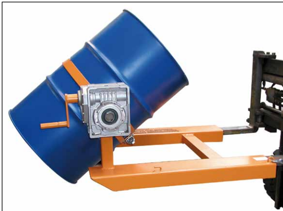
Typ FD/HK
