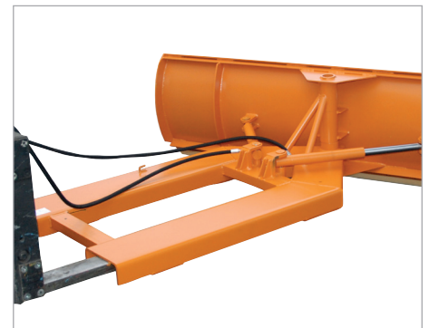
Hydraulische Schildverstellung
