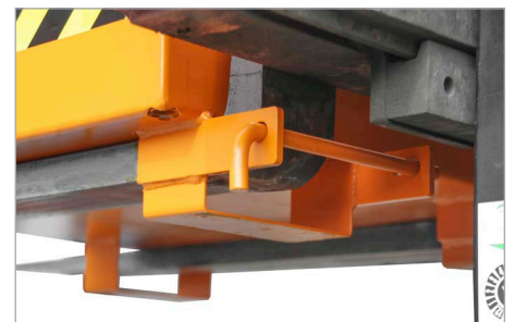
Bolzensicherung
