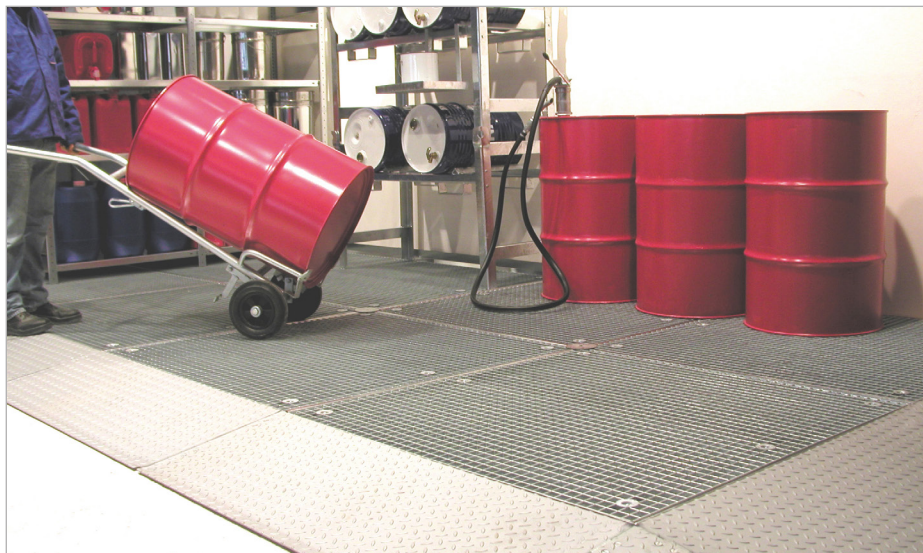
8 x BSW + 5 x AR + 1 x AE + 3 x KV + 10 x WV (options: diable à fûts FP-V, rayonnages à fûts FR)
