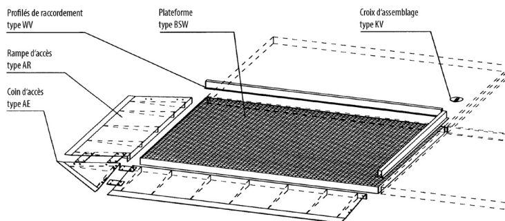
8 x BSW + 5 x AR + 1 x AE + 3 x KV + 10 x WV (options: palettes à fûts FP-2, rayonnages à fûts FR)
